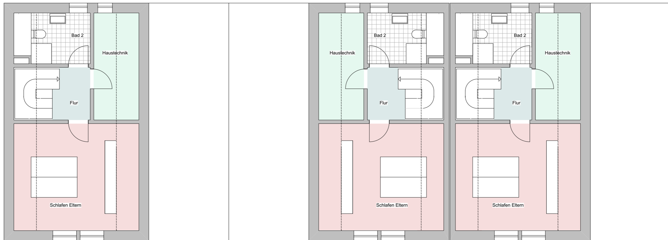
Dachgeschoss
